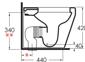
vaso tulip one installato su vecchio impianto tulip one wc old installation
