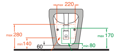
bidet tulip one installato su vecchio impianto tulip one bidet old installation
