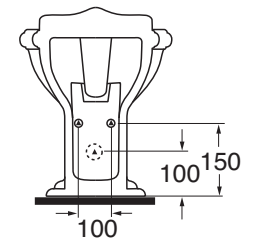
bidet tulip one installato su vecchio impianto tulip one bidet old installation
